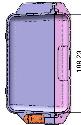
剖面 A-A
