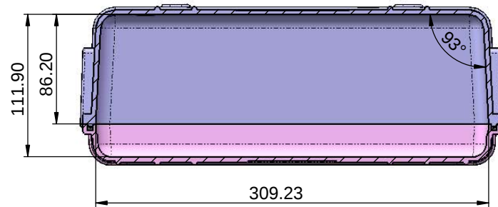
剖面 B-B
