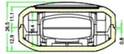
SEC A-A
